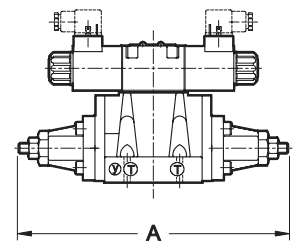
E*P4-S*/C
