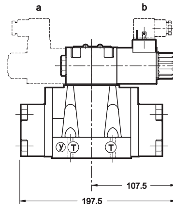
E4P4-TA E4P4-*TA
