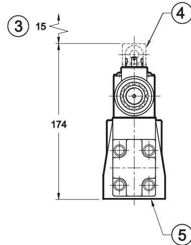
E4P4-TA E4P4-*TA
